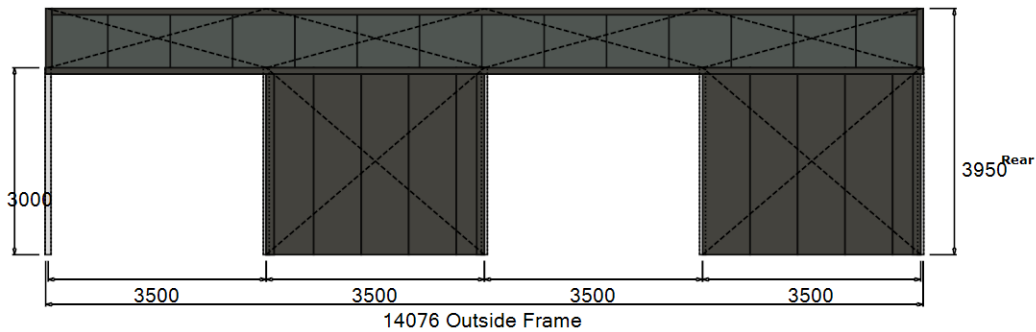
Right Elevation
